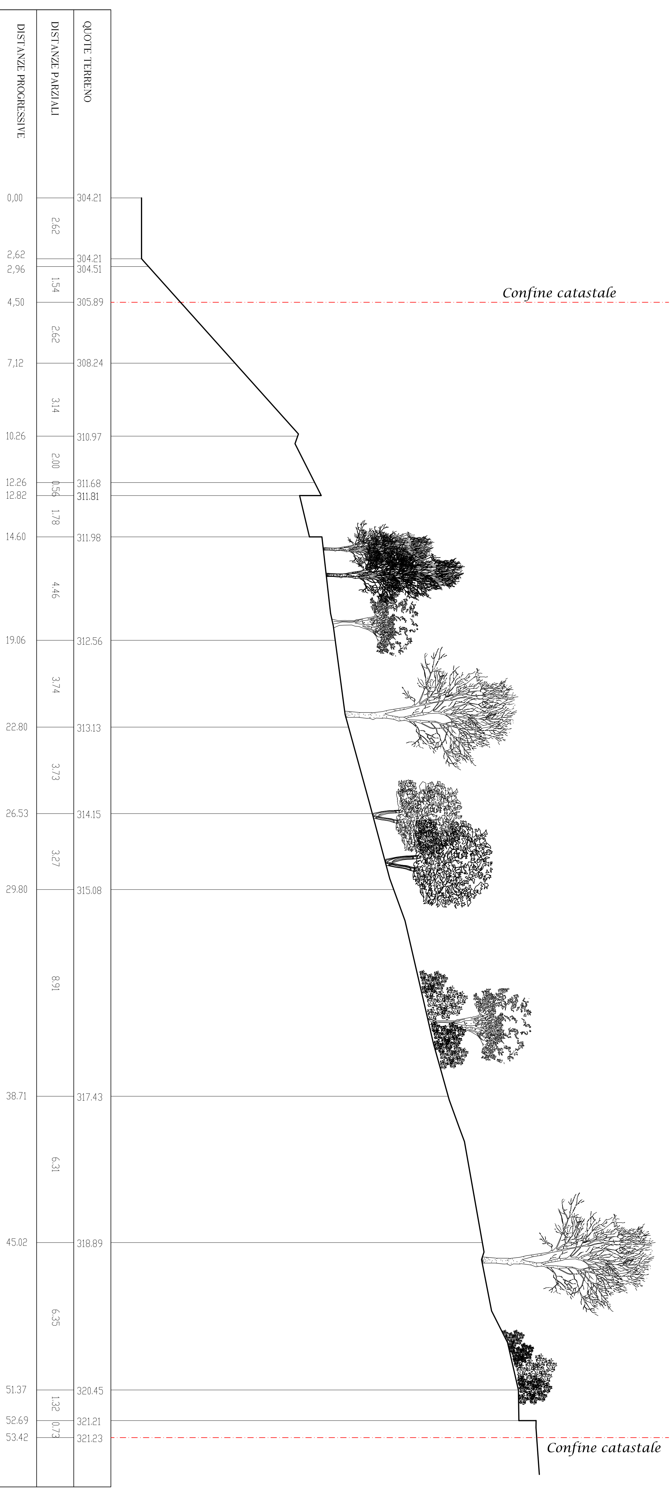
SEZIONE B-B'
