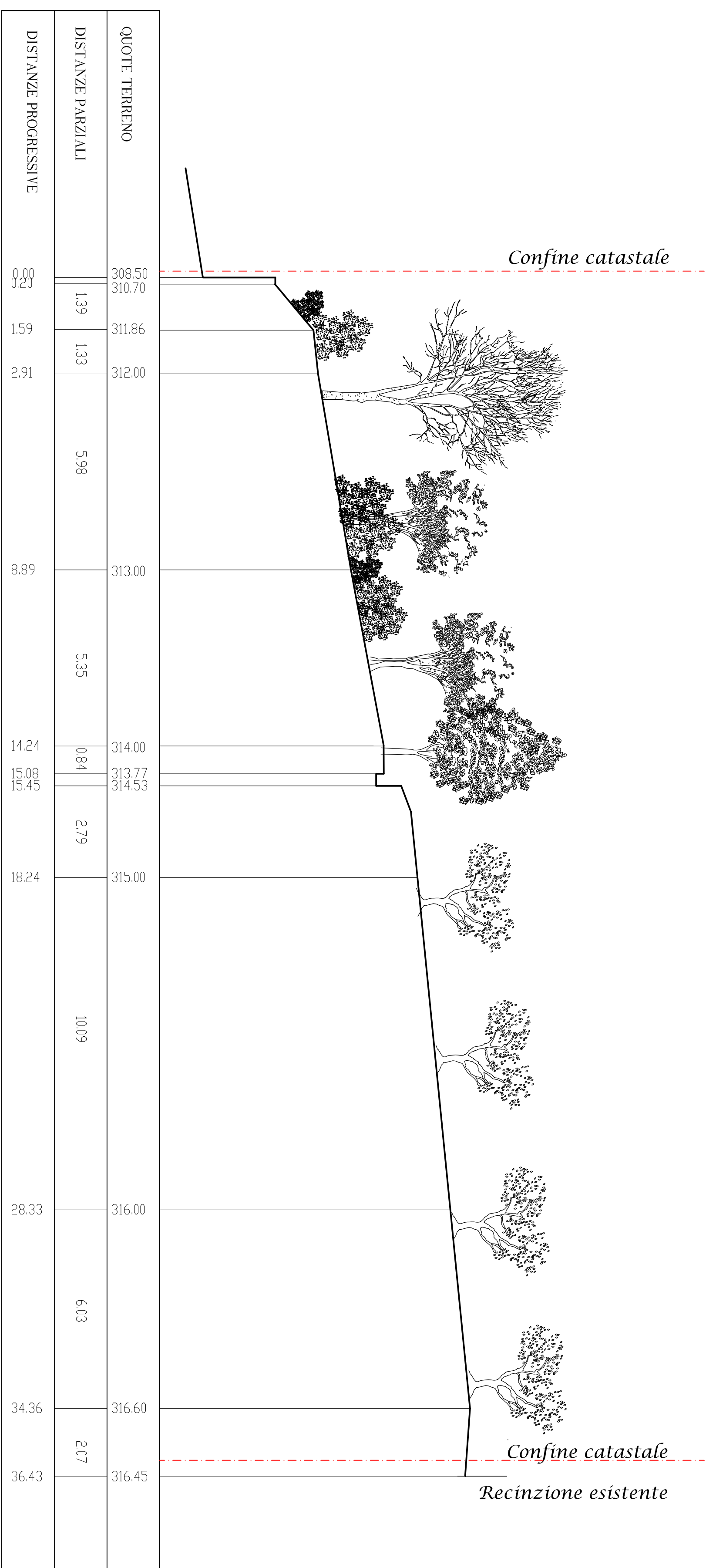
SEZIONE B-B'
