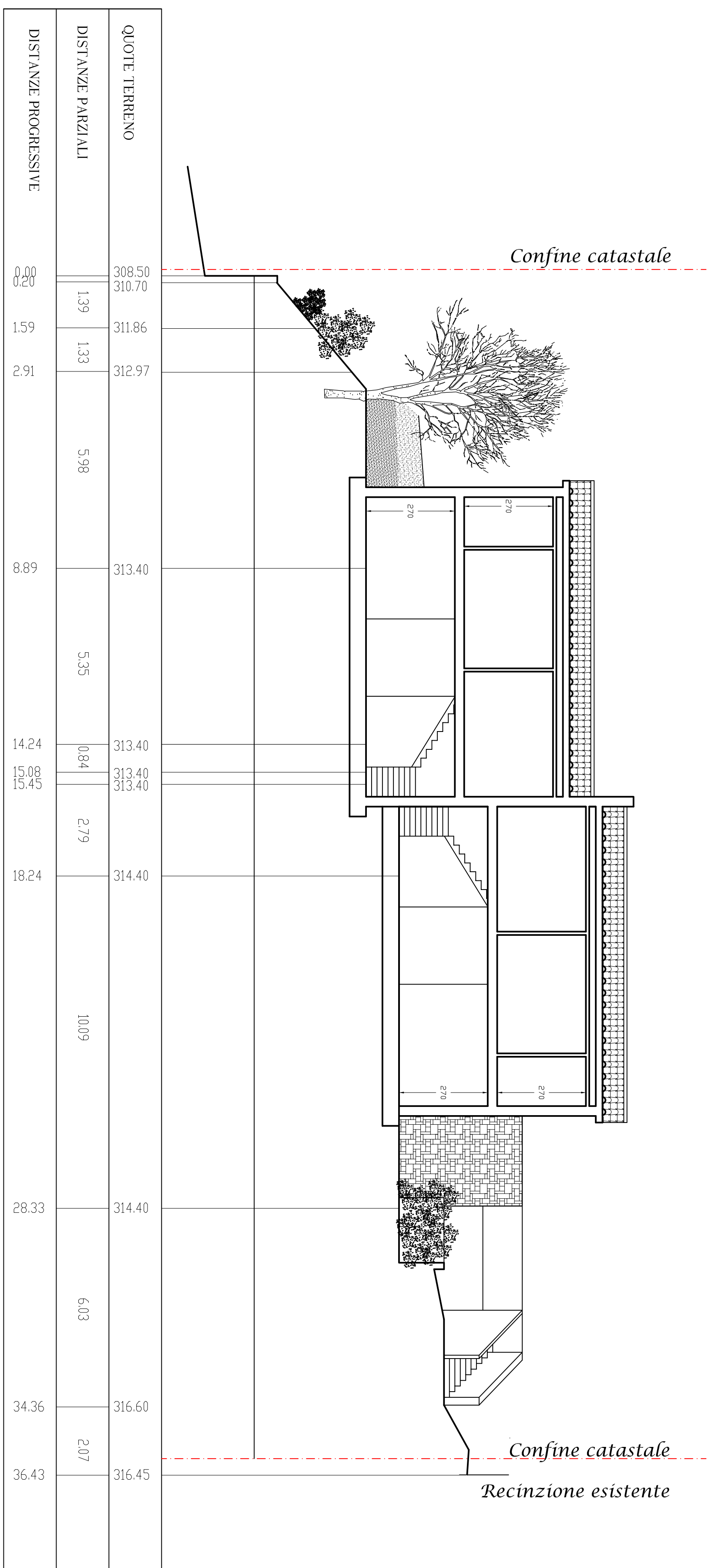
SEZIONE B-B'
