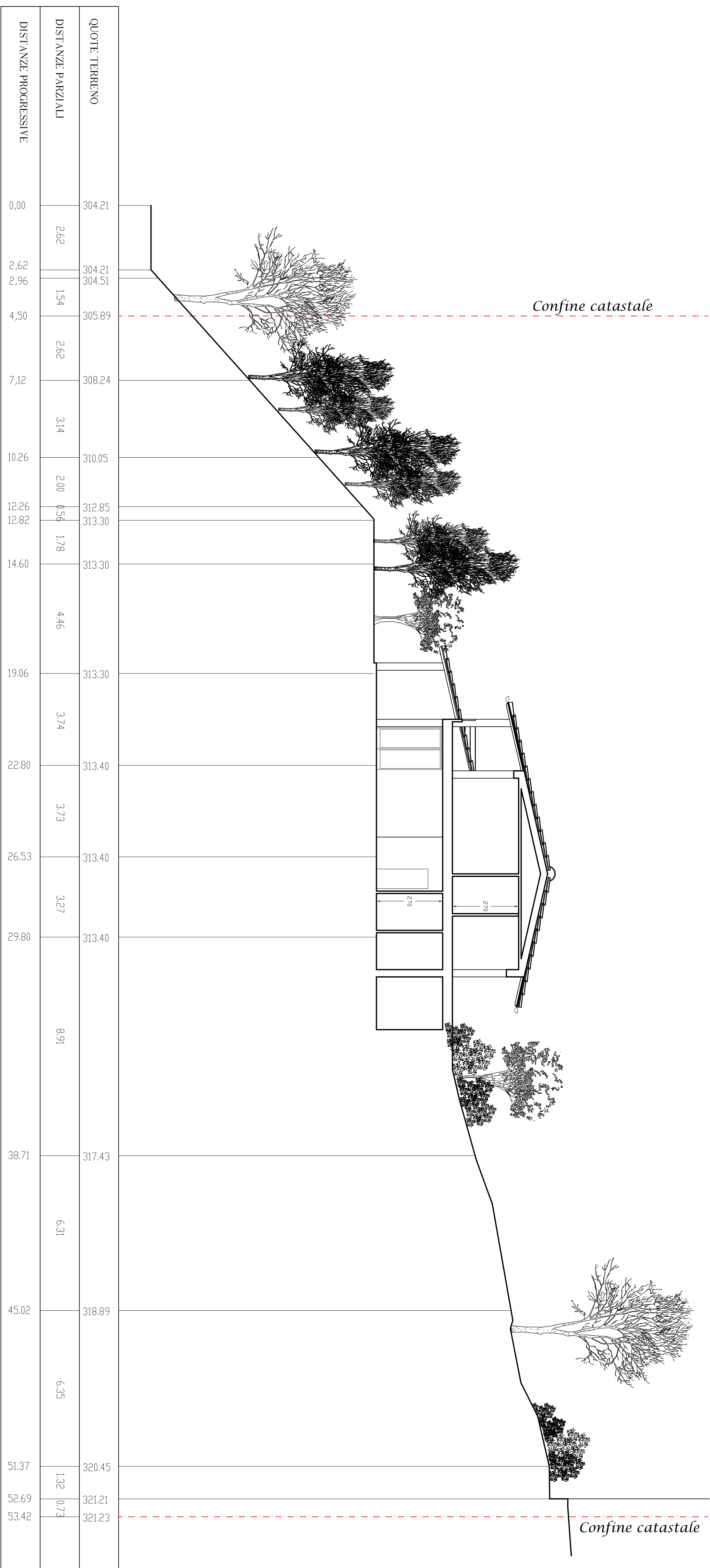
SEZIONE B-B*
