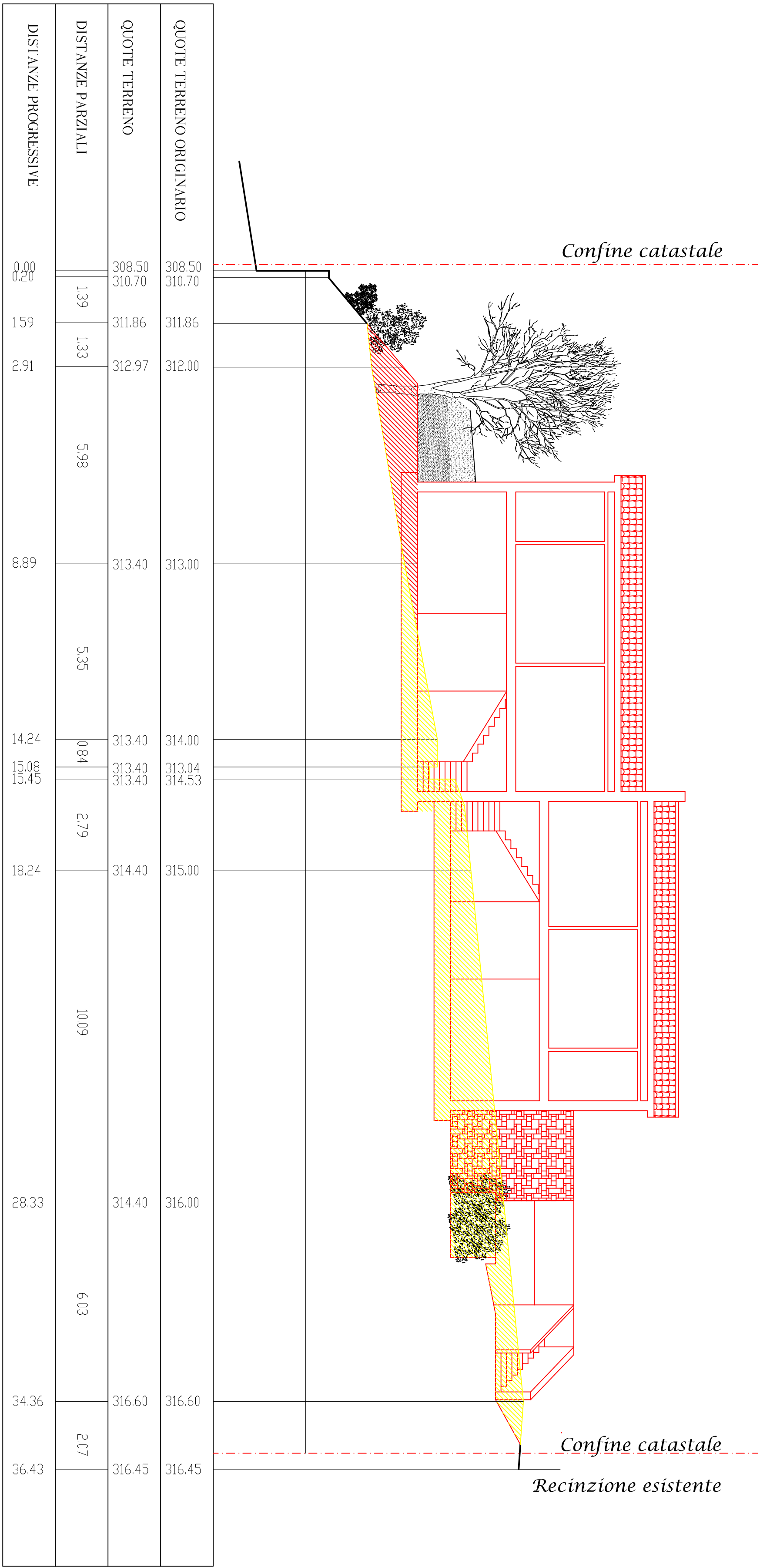
SEZIONE B-B'
