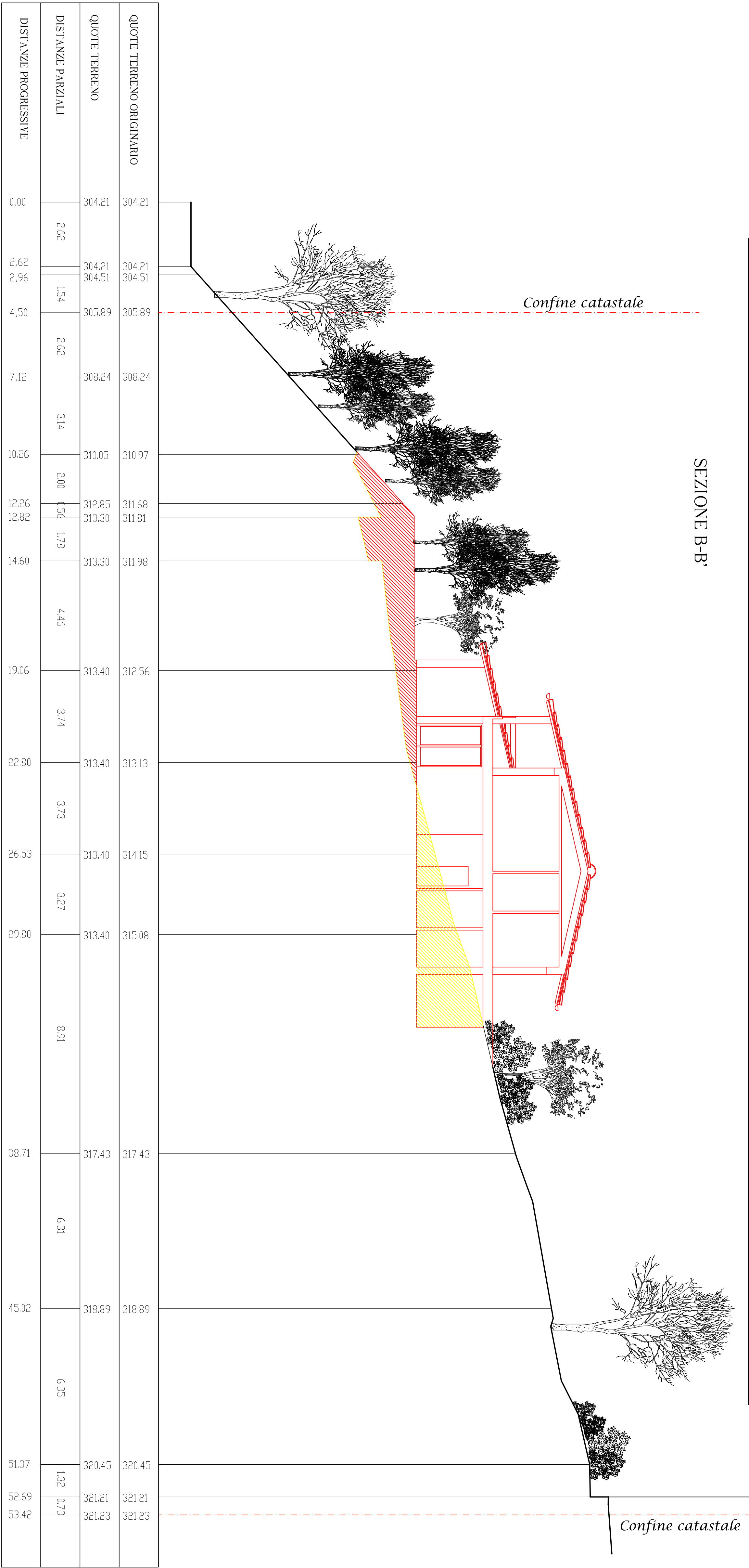
SEZIONE B-B'
